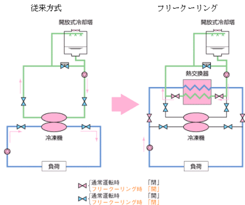
図1 フリークーリング制御へのリニューアルイメージ
